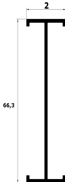
15346 REDUCTOR VIDRIO
