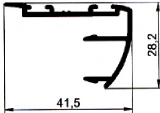
15421 CRUCE HOJAS
