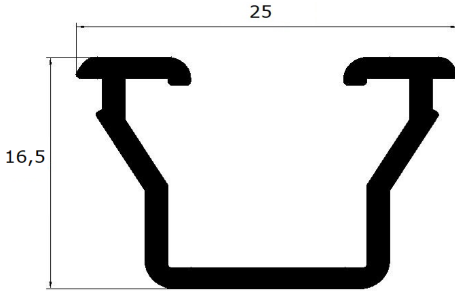
15346 REDUCTOR VIDRIO
