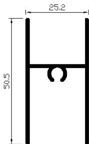
15325 TRAVESAÑO HOJA
