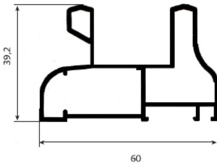
15410 MARCO DE 60
